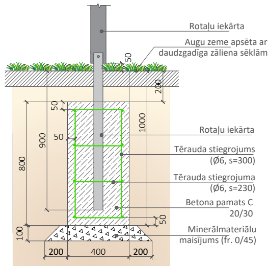
PRINCIPIĀLS ROTAĻU IEKĀRTAS STIPRINĀJUMA MEZGLS M 1:25
