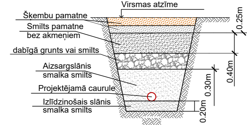
Tranšejas aizbēršanas shēma ar bruģa segumu
