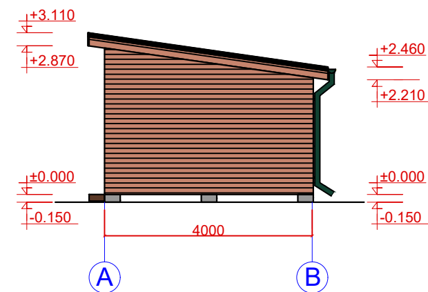
Fasāde asīs A-B M 1:100
