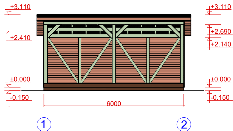
Fasāde asīs 1-2 M 1:100
