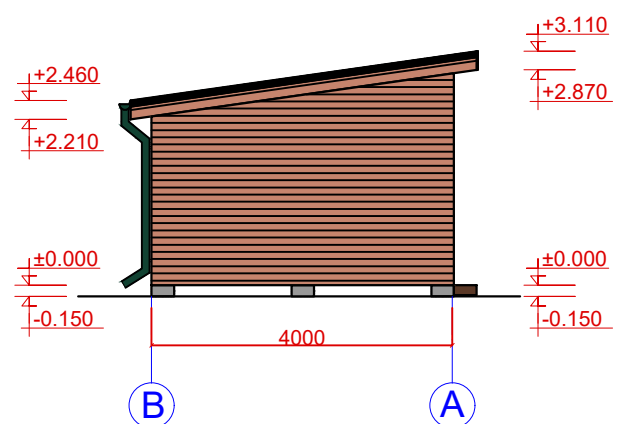
Fasāde asīs B-A M 1:100
